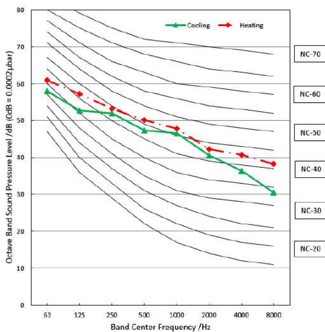
MOX230-12HFN8-QRD0W(GA)
