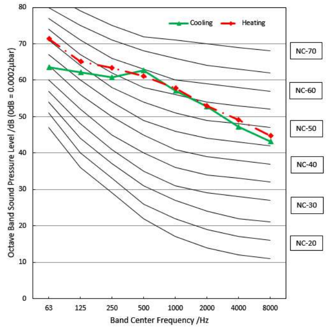
MOE30U-55HFN8-RRD0W(GA)
